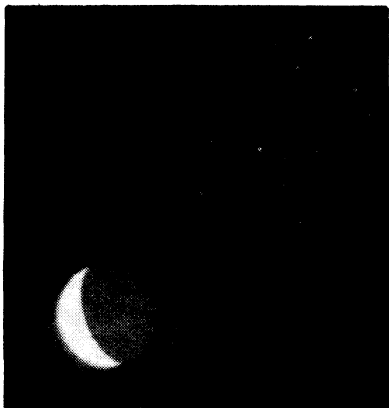
Рис. 24. Соединение Луны и Плеяд 27 июля 1935 г. Объектив Фойхтлендера (см. подпись к рис. 23). Пластинка «Опта», выдержка 1 мин. (увеличение 2,3×). Снимок Ж. де Вокулера.
