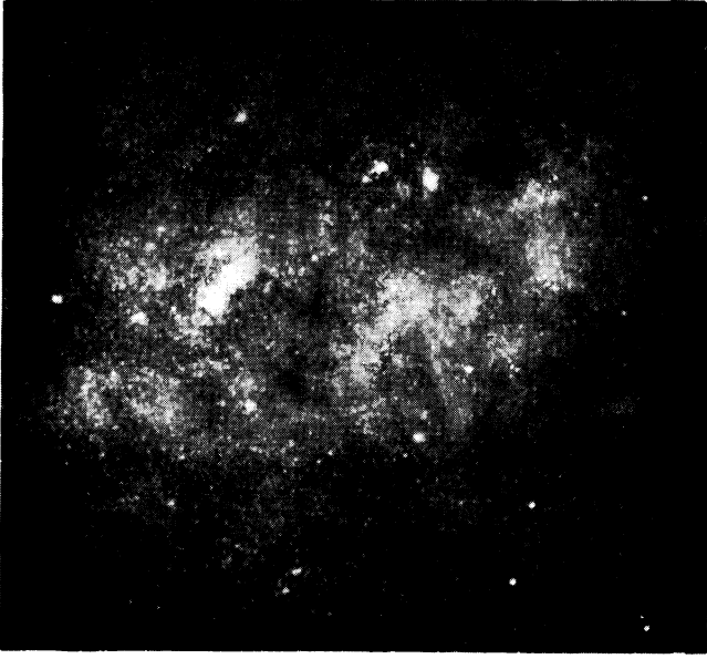
Фото III. Млечный Путь в Стрельце. Фотография вблизи южного горизонта Парижа показывает влияние атмосферного поглощения. Объектив «Стилор» Руссела с фокусным расстоянием 210 мм и светосилой 1/4,5, пластинка «Суперфугур», выдержка 1 час 5 мин.
