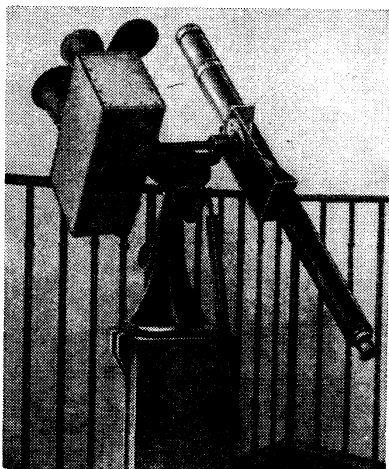
Рис. 19. Маленький фотографический экваториал на литом штативе с двумя спаренными камерами среднего фокусного расстояния, снабженными объективами «Стилор» Руссела с f = 210 мм и светосилой 1/4,5 и «Тессар» Цейсса с f = 250 мм и светосилой 1/3,5 . Телескоп-гид D = 60 мм (переделанная земная подзорная труба). Винт вращения часового круга управляется от руки.
