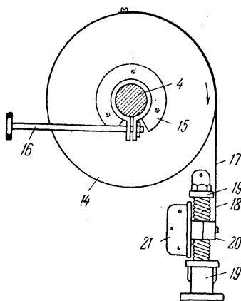
Рис. 516. Ведущий круг.
