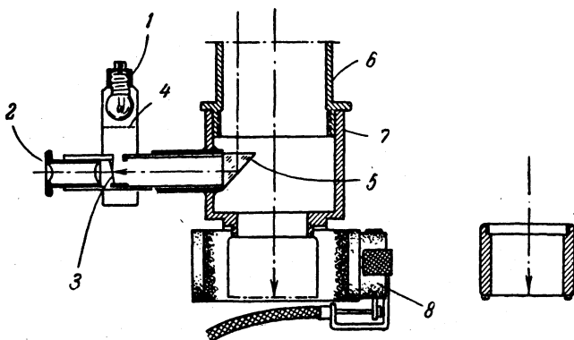
Рис. 44. Адаптер для малоформатной фокальной камеры с приспособлением для гидирования телескопа Кассегрена.
